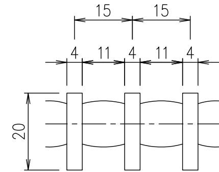
メインバーピッチ詳細図 S=1/1
