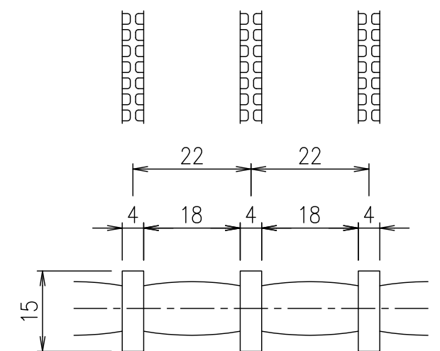
メンバーピッチ詳細図 S=1/1
