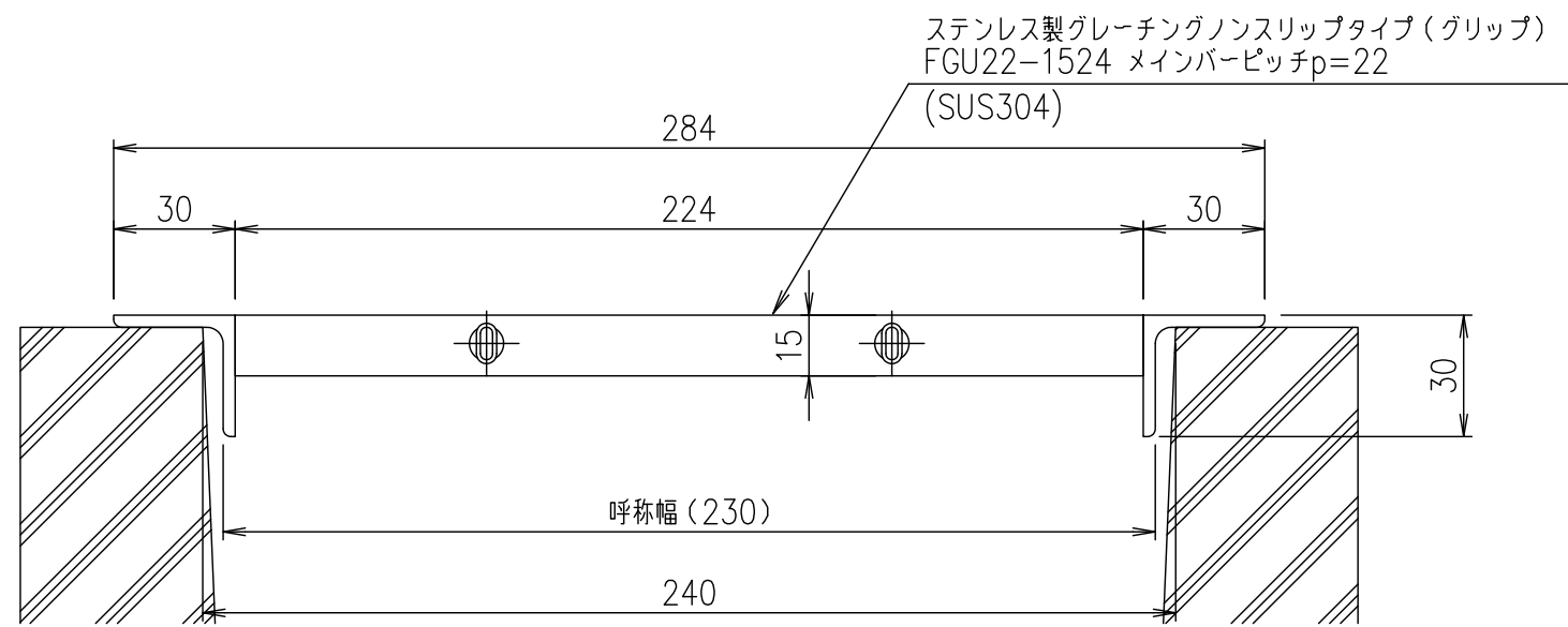
断面詳細図 S=1/2
