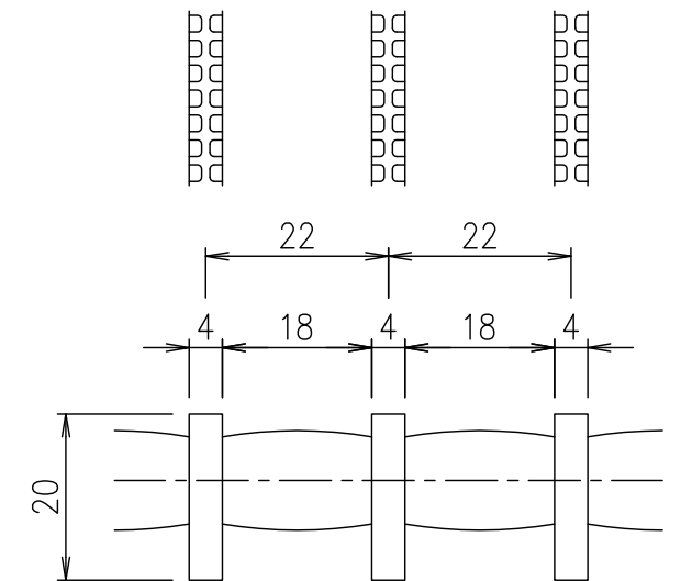
メンバーピッチ詳細図 S=1/1
