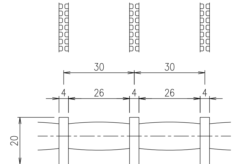
メンバーピッチ詳細図 S=1/1
