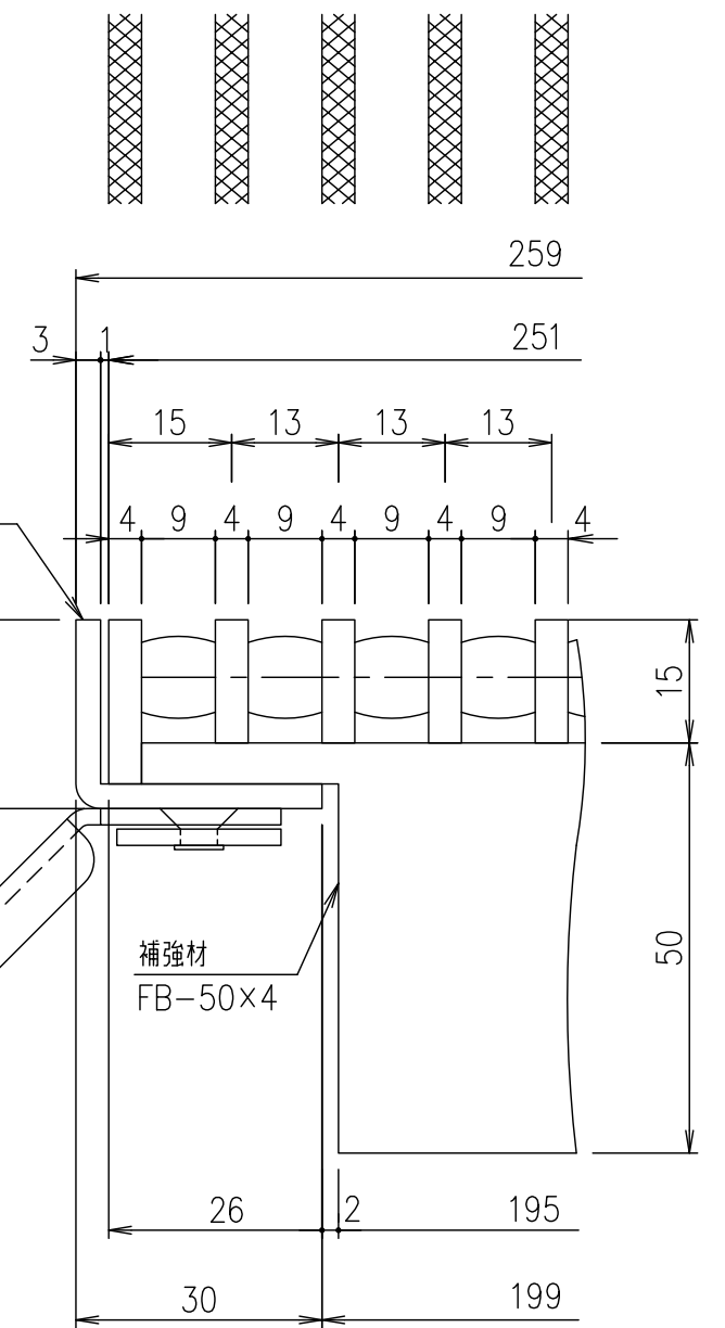
受枠断面・メインバーピッチ詳細図 S=1/1
