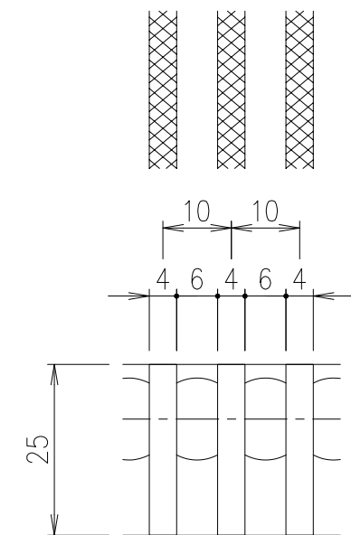
メンバーピッチ詳細図 S=1/1
