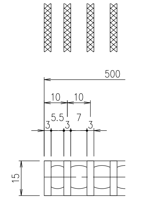
メンバーピッチ詳細図 S=1/1
