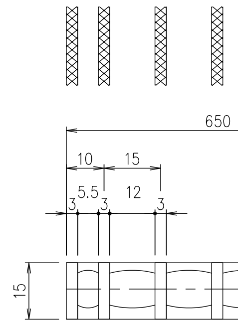
メンバーピッチ詳細図 S=1/1
