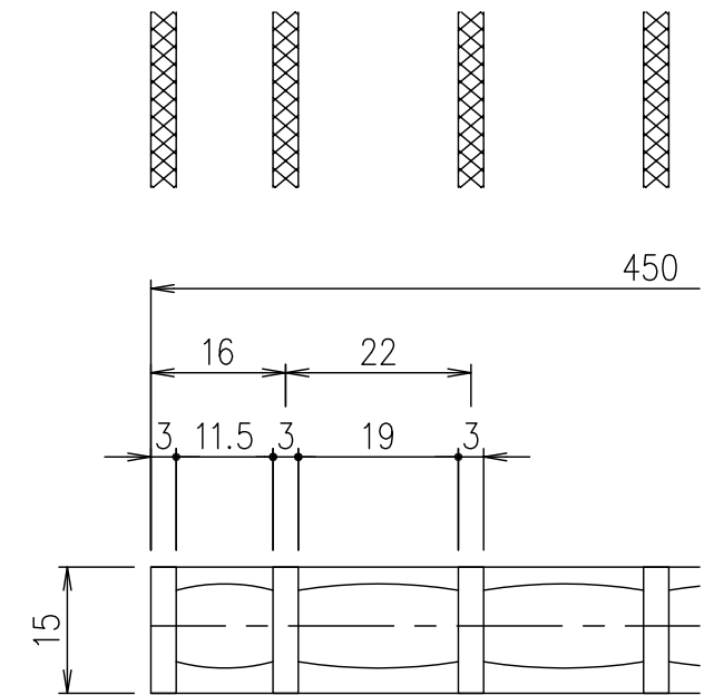
メンバーピッチ詳細図 S=1/1
