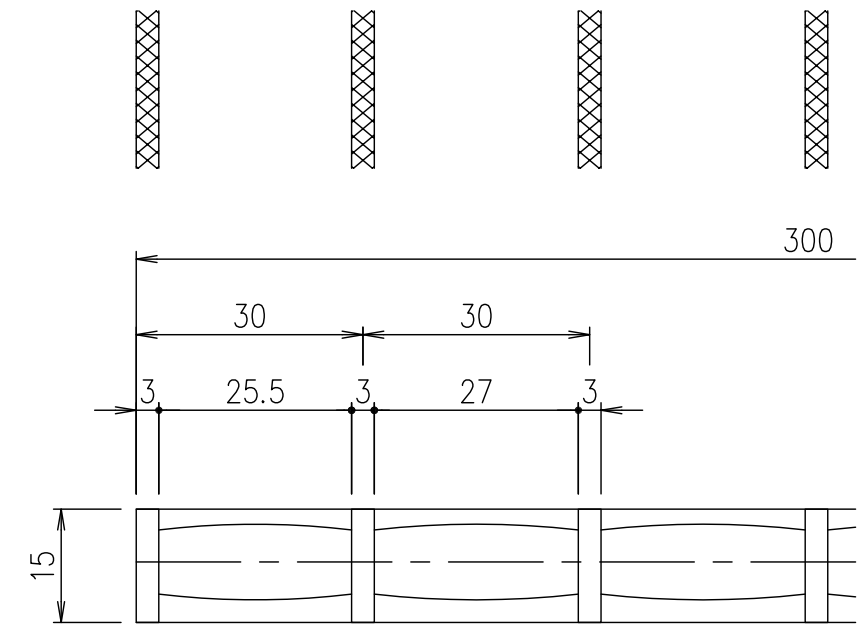
メンバーピッチ詳細図 S=1/1
