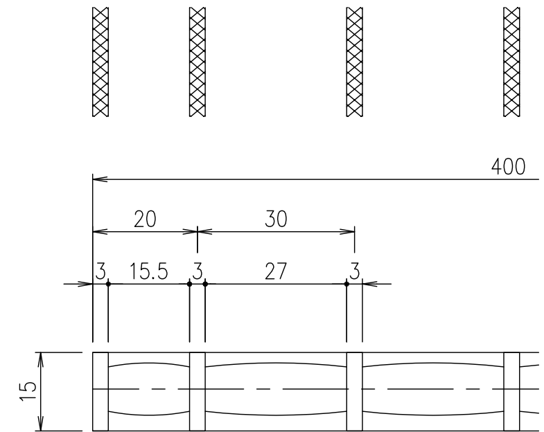
メンバーピッチ詳細図 S=1/1
