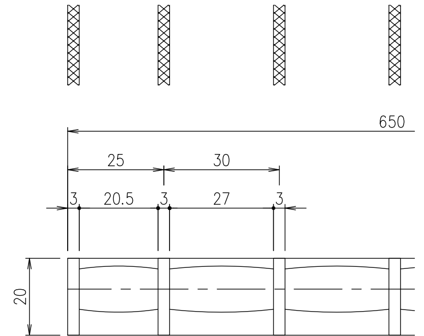
メンバーピッチ詳細図 S=1/1
