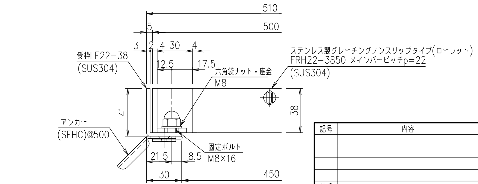
受枠断面詳細図 S=1/2
