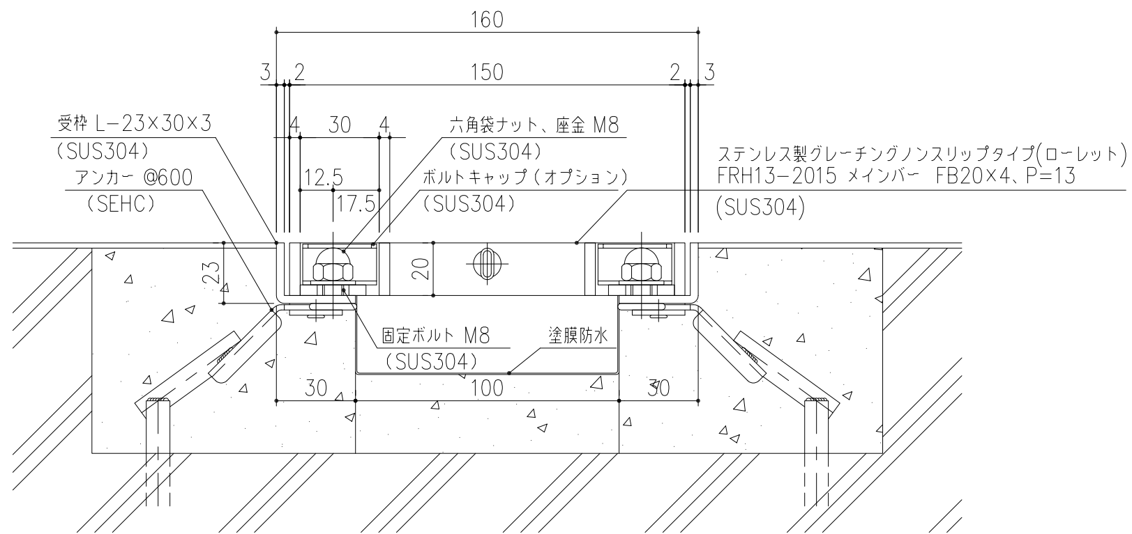
受枠断面詳細図 S=1/2
