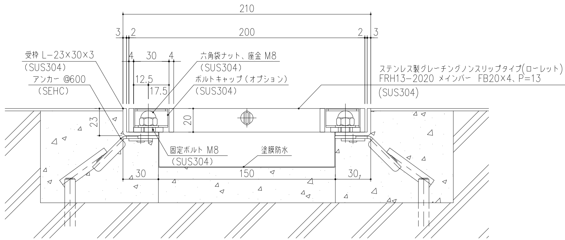
受枠断面詳細図 S=1/2
