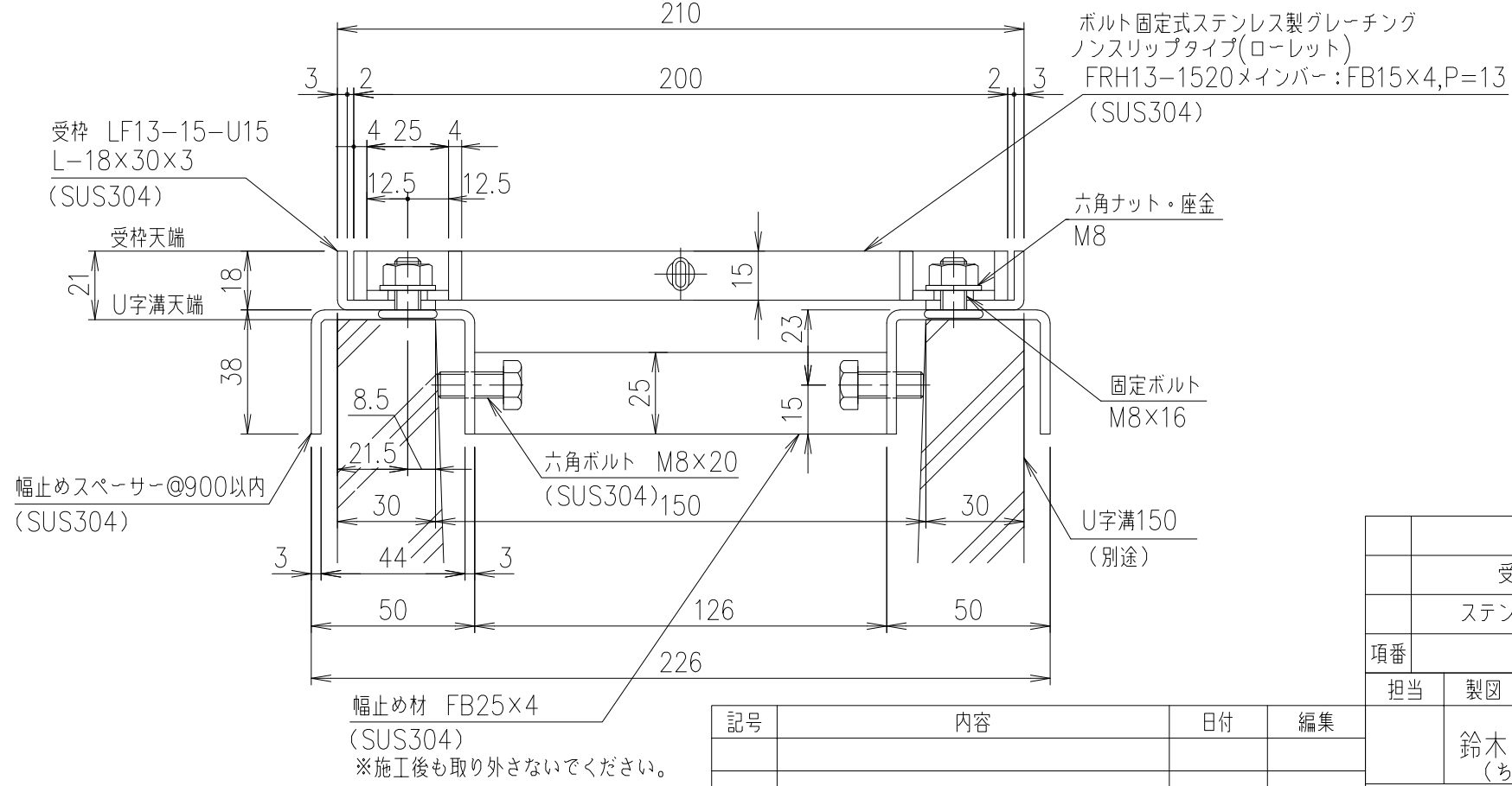
断面詳細図 S=1/2
