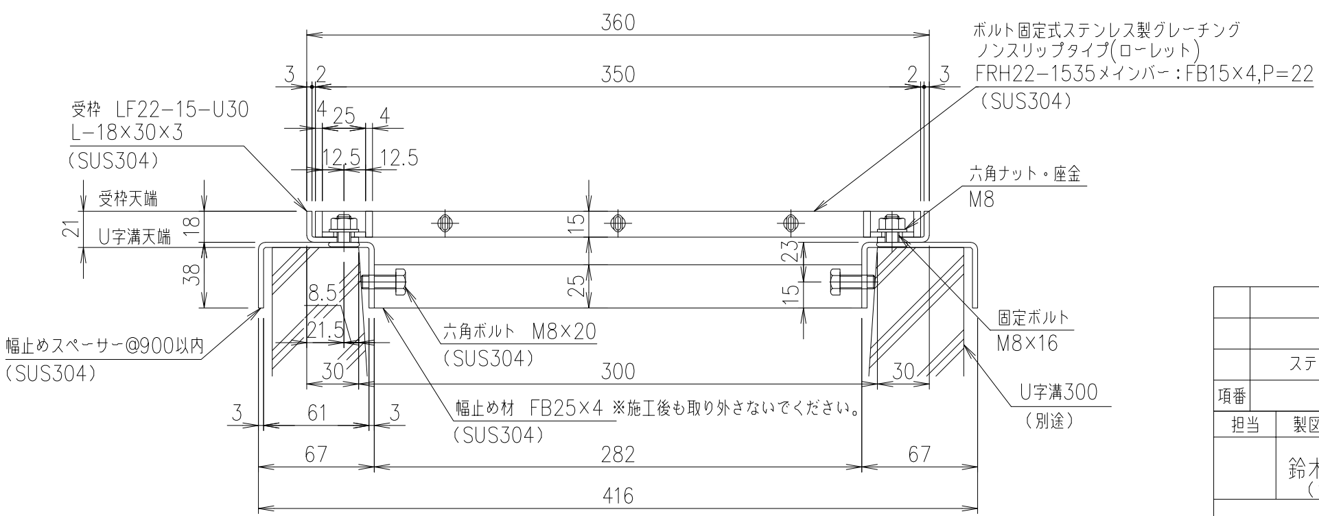
断面詳細図 S=1/3
