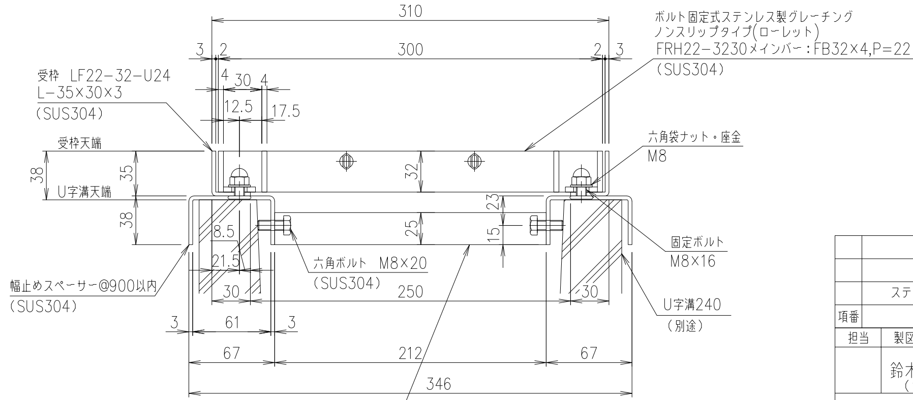
断面詳細図 S=1/3
