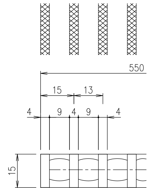
メンバーピッチ詳細図 S=1/1
