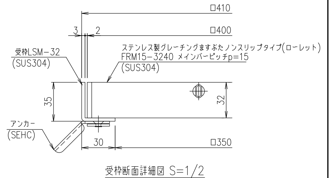
メインバーピッチ詳細図 S=1/1
