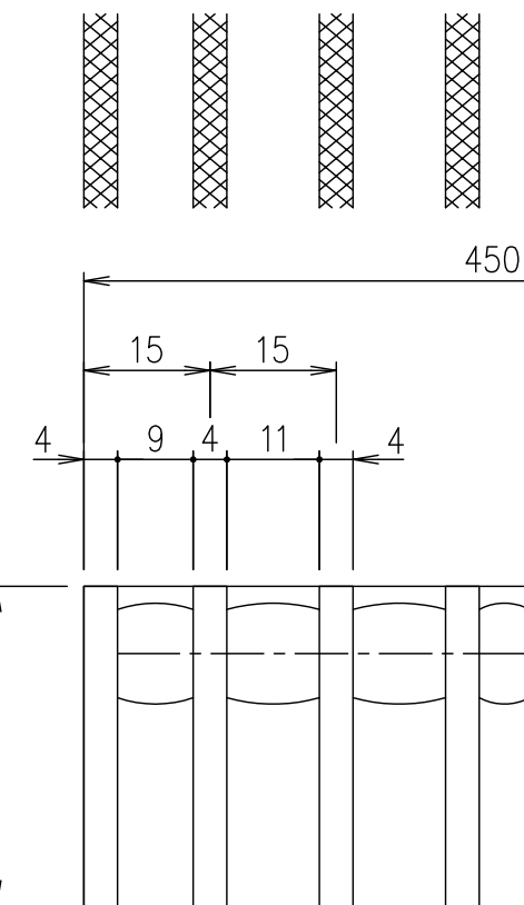
メインバーピッチ詳細図 S=1/1
