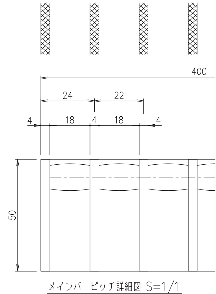
受枠LSM-50 (SUS304) ステンレス製グレーチングますぶたノンスリップタイプ(ローレット) FRM22-5040 メインバーピッチ p=22 (SUS304) アンカー (SEHC) □410 □400 53 50 30 □350
