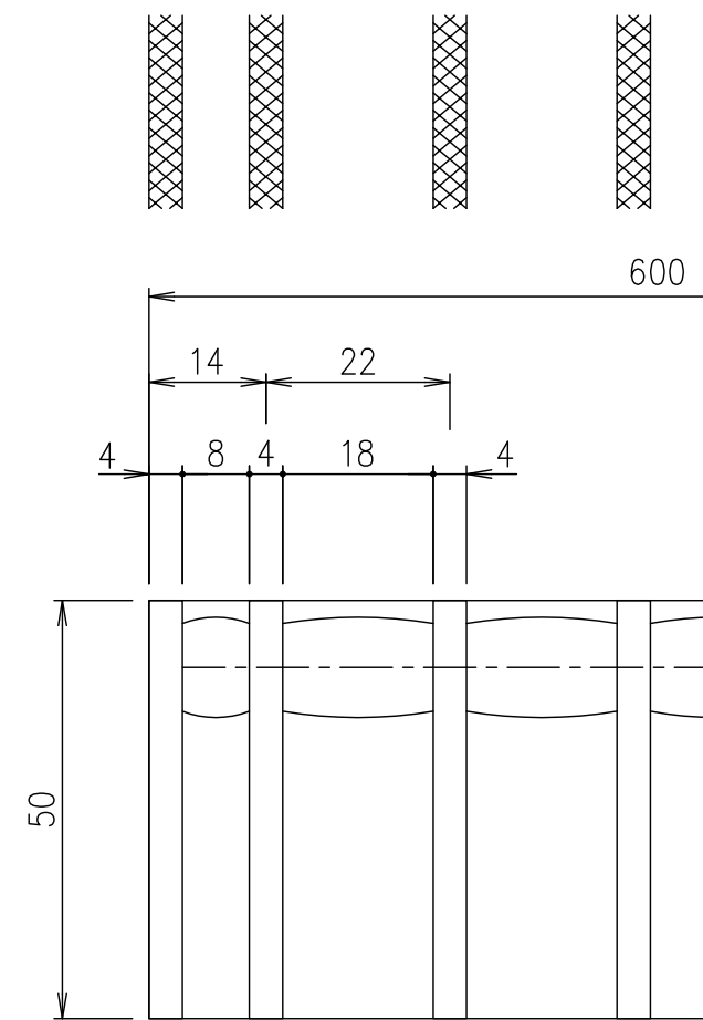
メインバーピッチ詳細図 S=1/1
