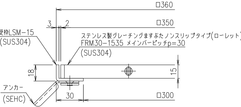
受枠断面詳細図 S=1/2
