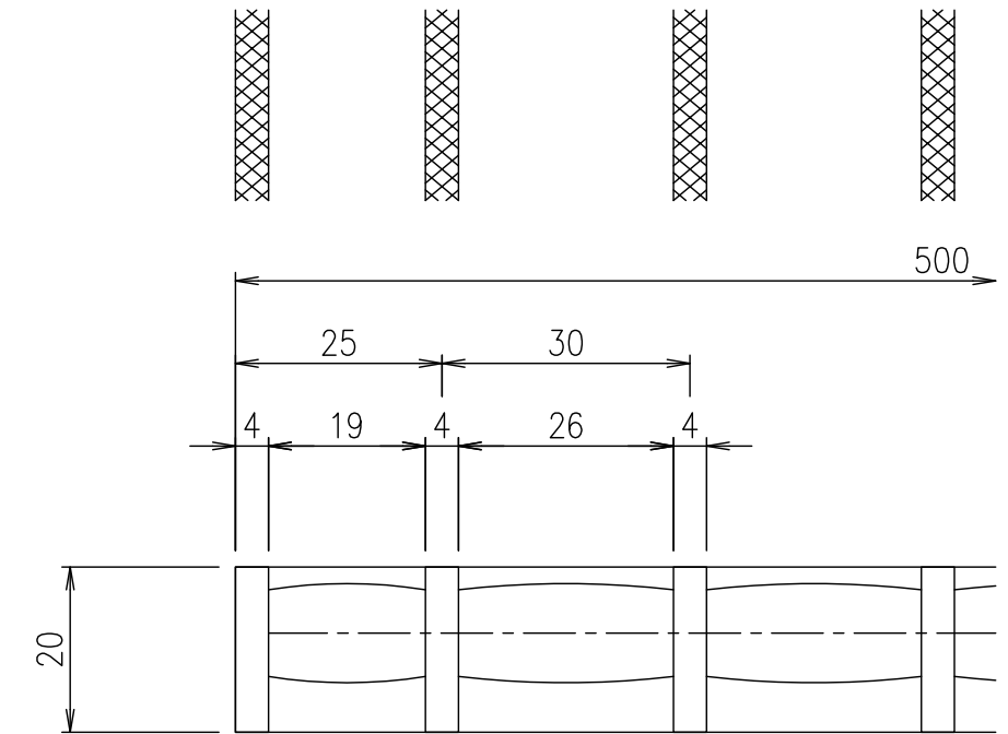
メンバーピッチ詳細図 S=1/1
