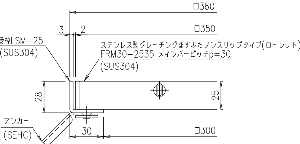
受枠断面詳細図 S=1/2
