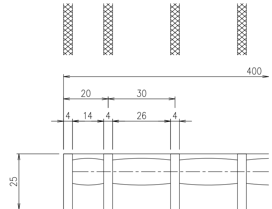
メンバーピッチ詳細図 S=1/1
