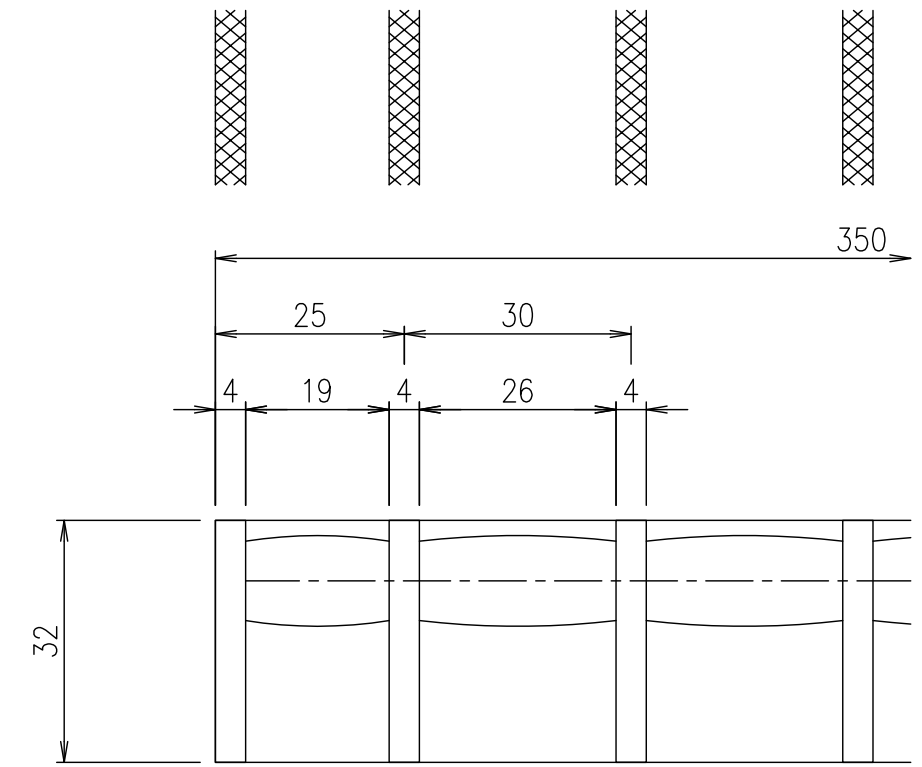
メンバーピッチ詳細図 S=1/1
