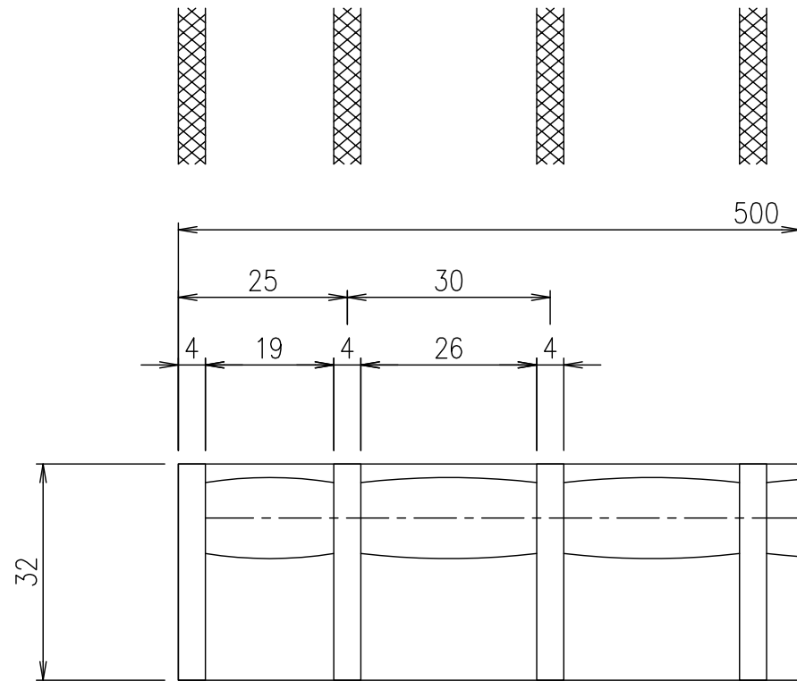
メンバーピッチ詳細図 S=1/1
