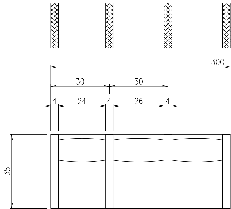
メンバーピッチ詳細図 S=1/1
