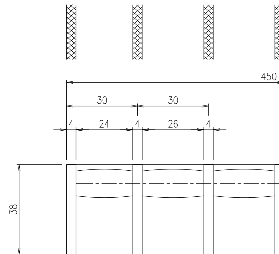
メインバーピッチ詳細図 S=1/1
