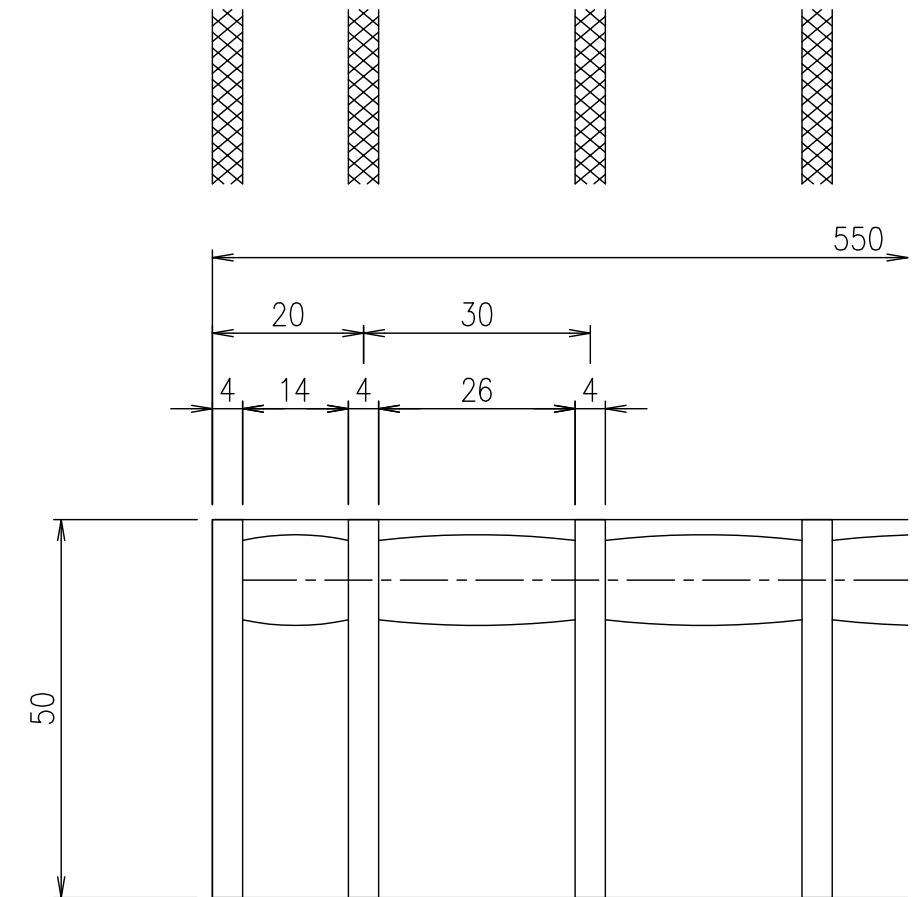
メインバーピッチ詳細図 S=1/1
