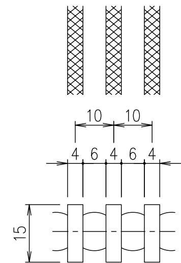
メンバーピッチ詳細図 S=1/1
