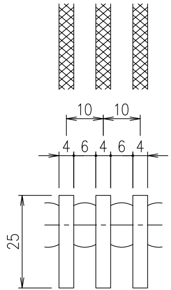
メインバーピッチ詳細図 S=1/1
