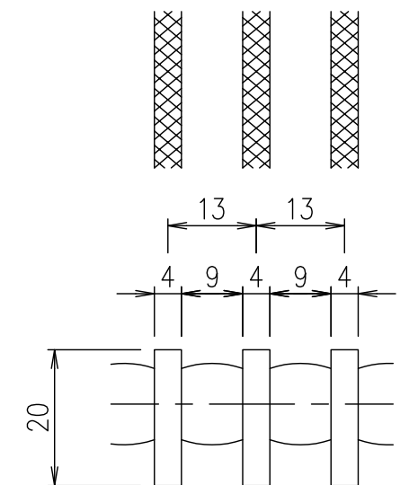
メンバーピッチ詳細図 S=1/1
