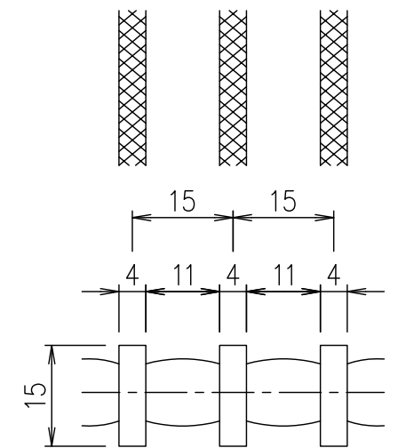
メンバーピッチ詳細図 S=1/1
