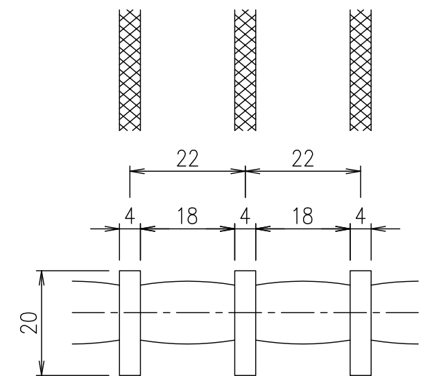
メンバーピッチ詳細図 S=1/1
