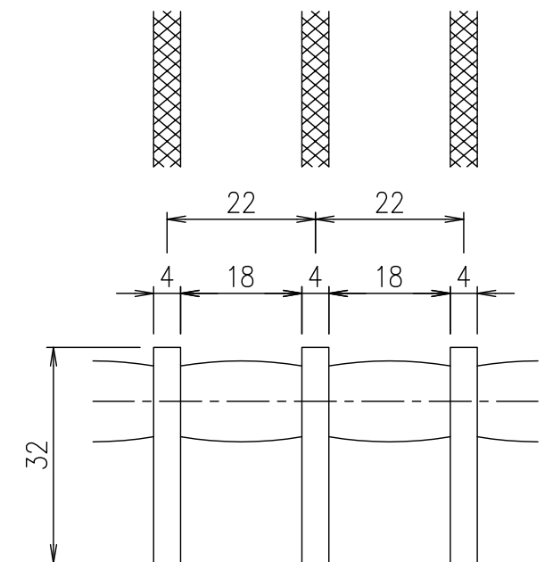
メンバーピッチ詳細図 S=1/1
