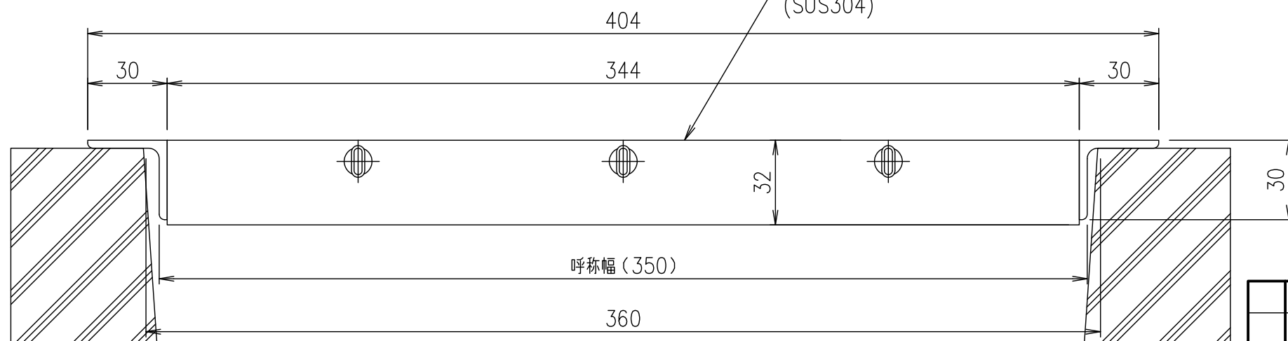
断面詳細図 S=1/2
