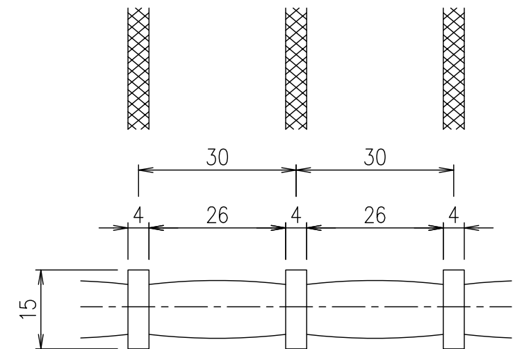
メンバーピッチ詳細図 S=1/1
