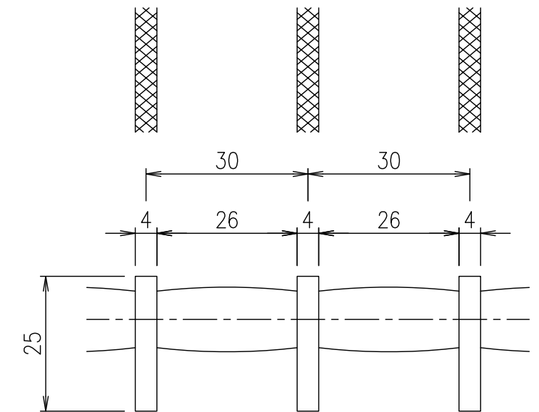
メンバーピッチ詳細図 S=1/1
