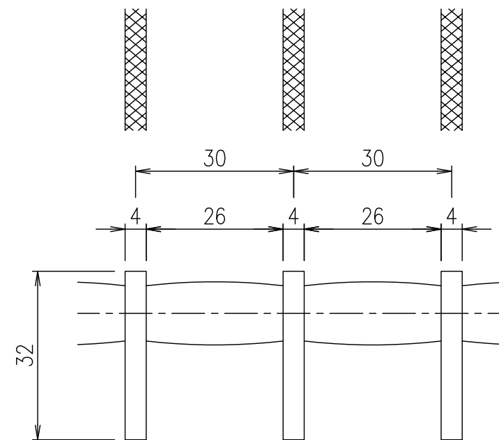
メインバーピッチ詳細図 S=1/1
