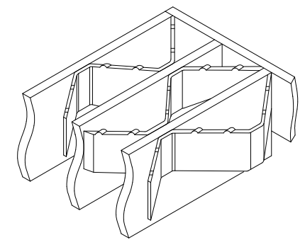
スベリ止め詳細図
