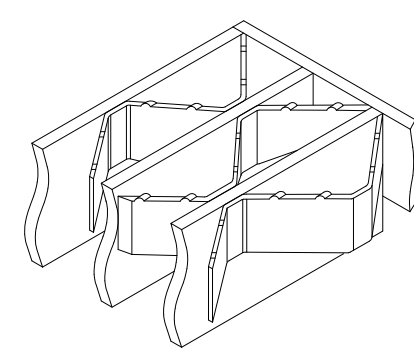
スベリ止め詳細図
