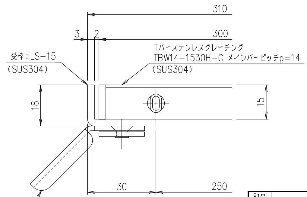
アンカー (SEHC) @500 受枠断面詳細図 S=1/1
