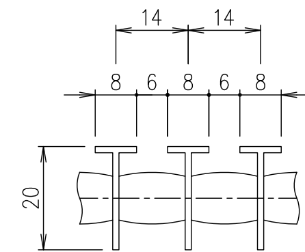
メンバーピッチ詳細図 S=1/1
