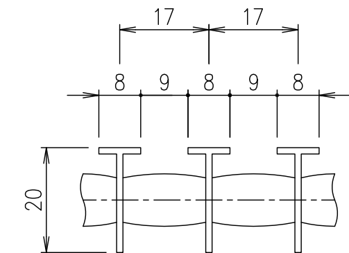
メンバーピッチ詳細図 S=1/1
