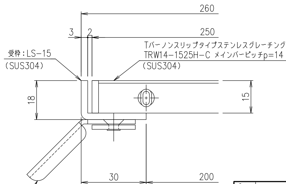
受枠断面詳細図 S=1/1
