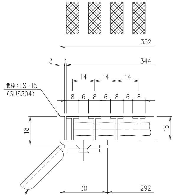
アンカー (SEHC) @500 受枠断面・メインバーピッチ詳細図 S=1/1
